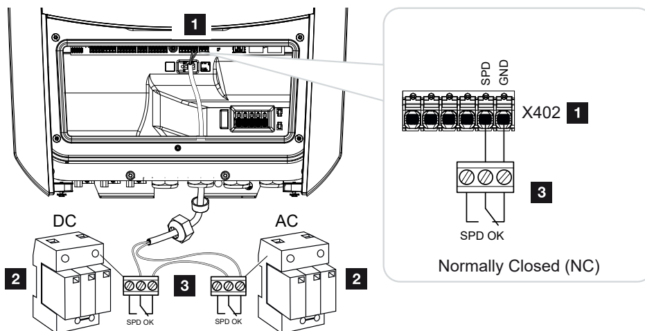
Fig. 1: Overspændingsbeskyttelse (SPD) som åbnekontakt
