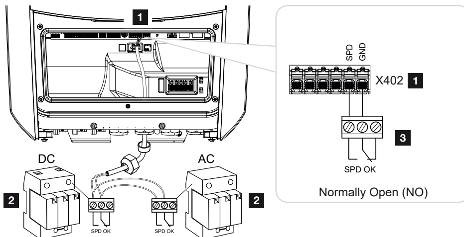
Fig. 2: Overspændingsbeskyttelse som sluttekontakt
