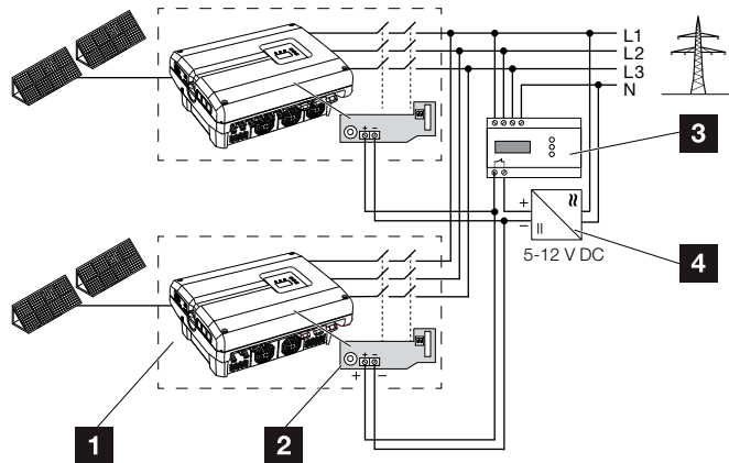
Kuva 25: Suojakatkaisijan toiminto
