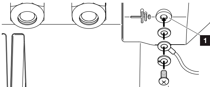
Kuva 24: Maakohtainen PE-liitäntä
