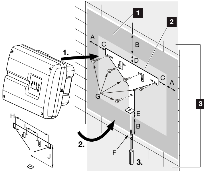
Kuva 19: Seinäasennus seinäkiinnikkeellä
