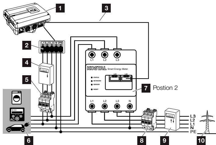
Kuva 66: Energiamittarin liitäntä
