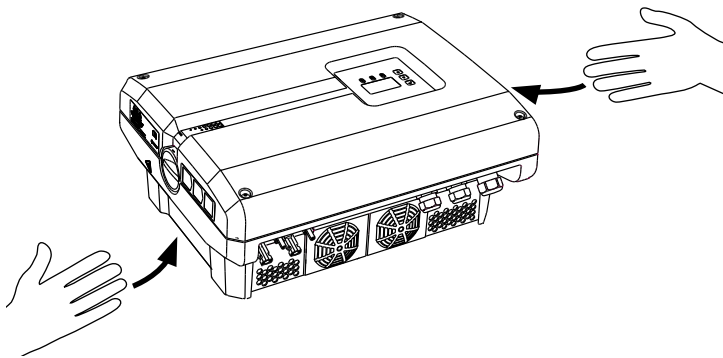
Kuva 17: Invertterin kädenpaikat
