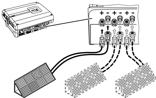
Kuva 30: DC-liitäntöjen yleisnäkymä
