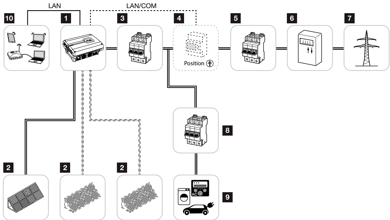
Kuva 8: 3-vaiheinen aurinkosähköjärjestelmä
