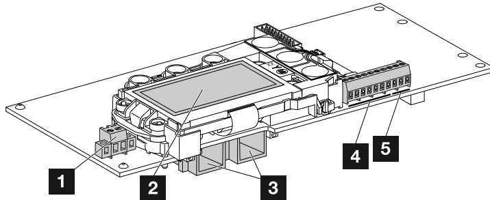
Kuva 14: Kommunikaatiokortin komponentit
