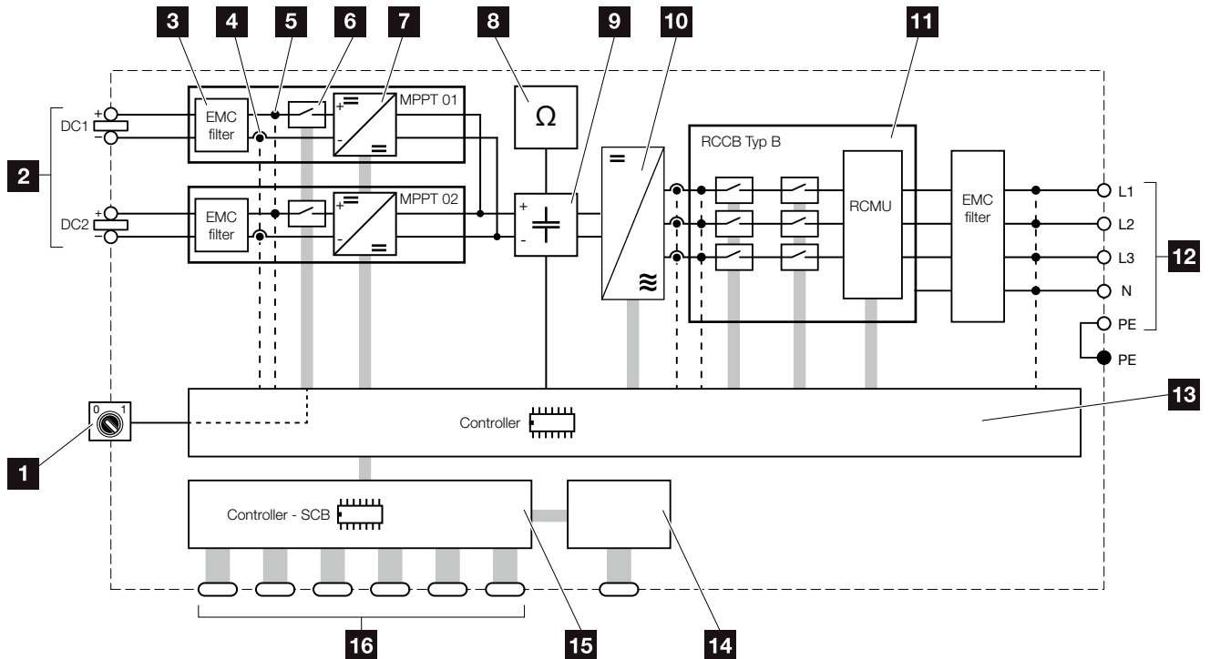
Bild 68: Blockkopplingsschema
