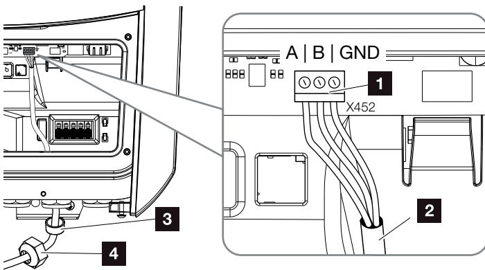
Bild 27: Ansluta digital energimätare (Modbus RTU)
