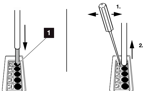
Bild 22: Fjäderbelastad kopplingsplint
