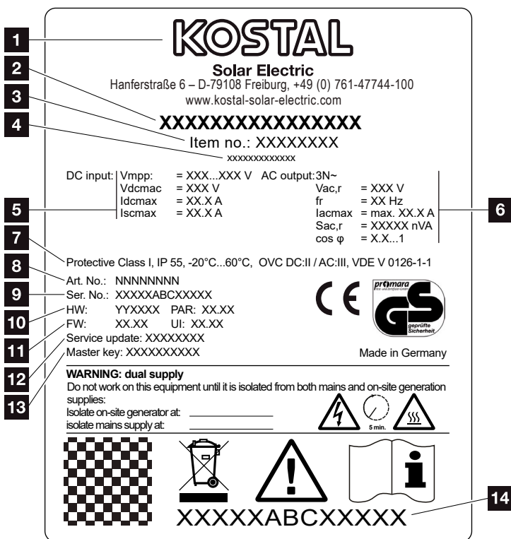
Bild 69: Typskylt
