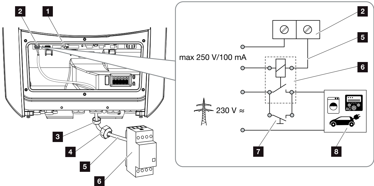
Bild 55: Elanslutning egenförbrukare
