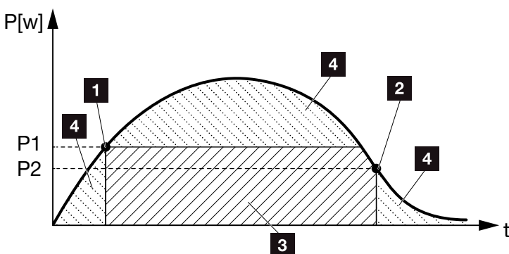
Bild 59: Kurva Egenförbrukning (funktion 2)
