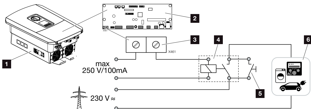
Bild 30: Anslutning av egenförbrukare
