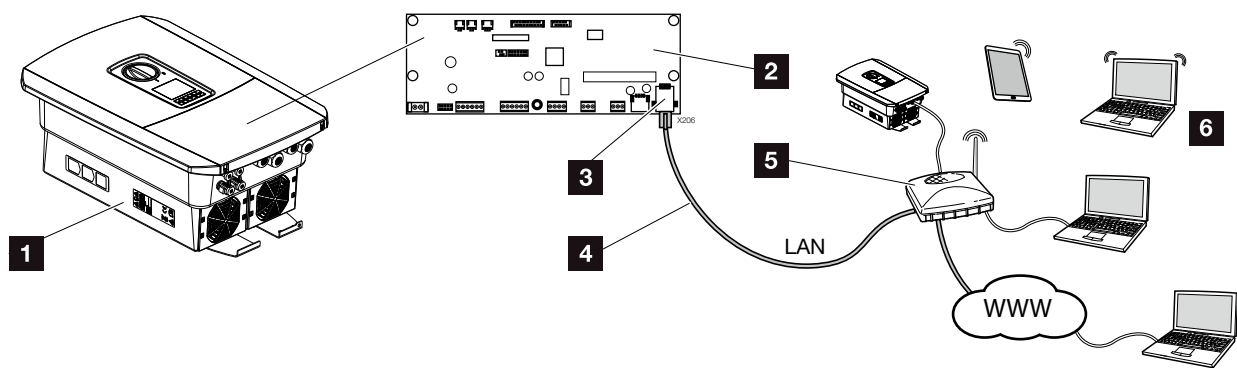
Bild 31: Anslutning av kommunikation
