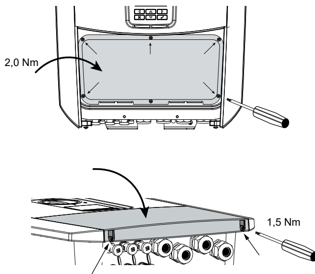
Bild 33: Stäng växelriktaren
