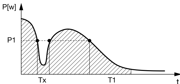
Bild 61: Kurva Fördröjning vid effektförlust / störning
