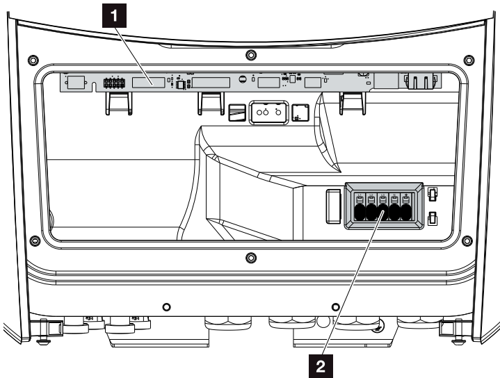
Bild 11: Växelriktare (insida)
