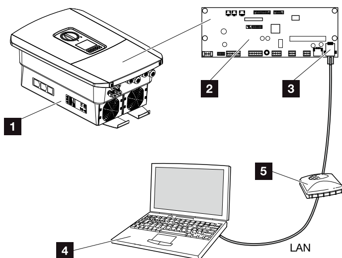
Bild 46: Anslut växelriktaren till datorn med Ethernet-kabeln
