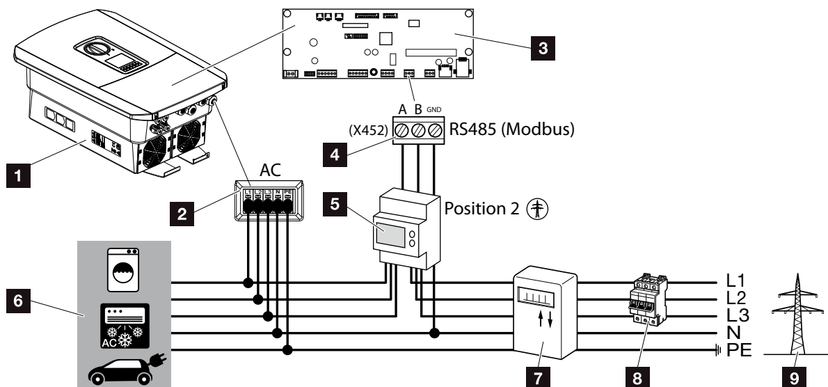
Bild 26: Anslutningsplan energimätare – nätanslutning (position 2)
