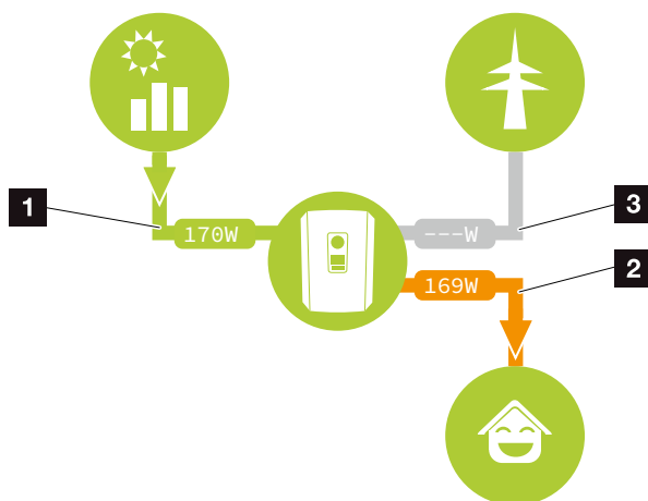
Bild 49: Energiflödesdiagram
