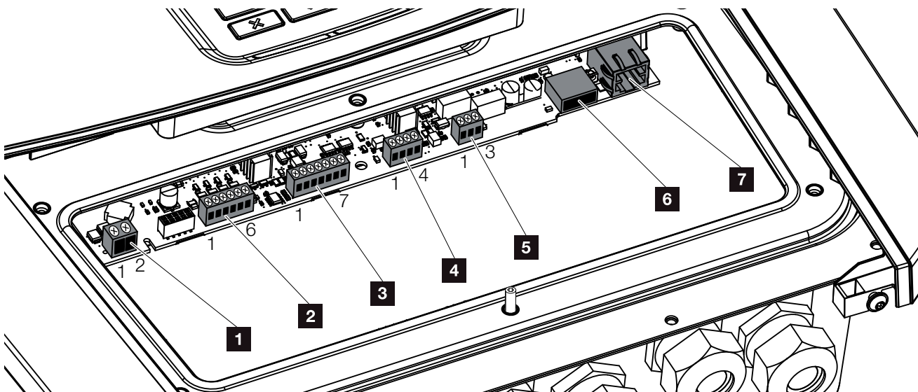
Bild 24: Smart Communication Board (SCB) – gränssnitt
