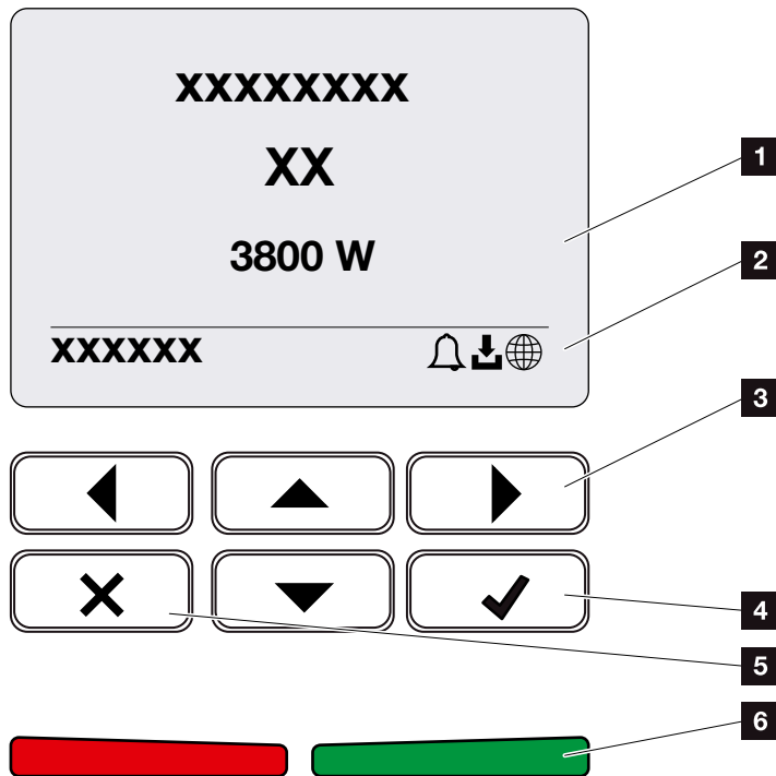
Bild 37: Manöverfält
