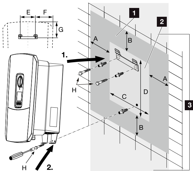
Bild 16: Väggmontering med hjälp av väggfäste
