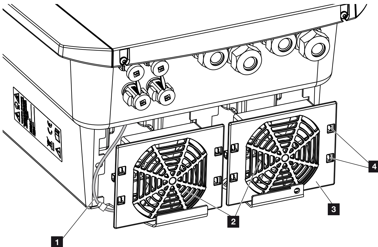
Bild 62: Översikt över fläktmontering
