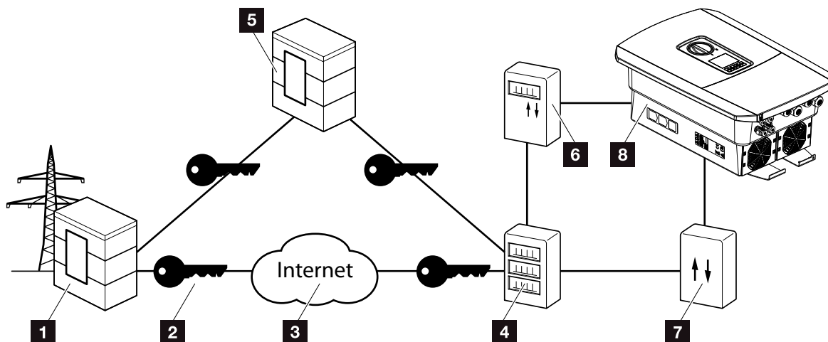
Bild 53: Anslutning av intelligenta mätsystem
