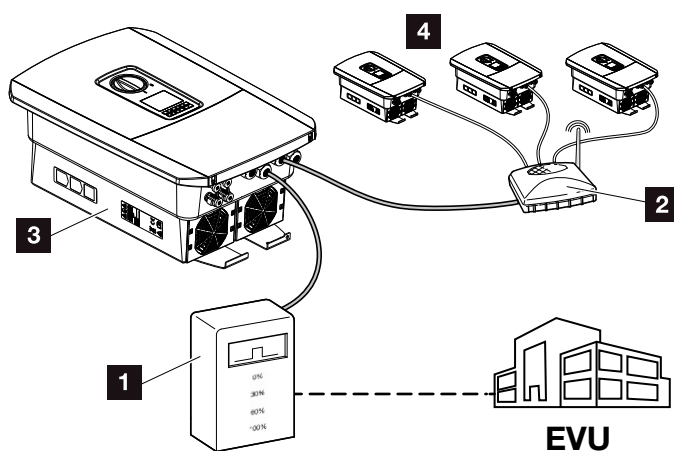
Bild 52: Växelriktare med rundstyrningsmottagare
