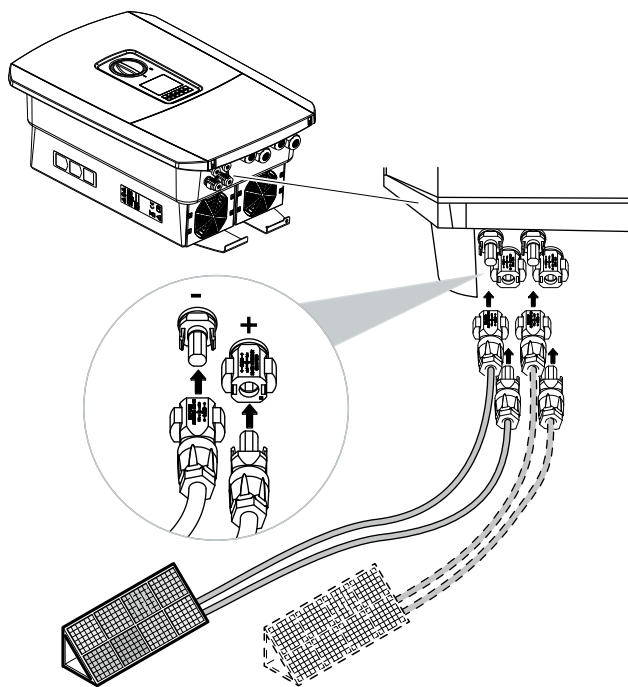
Bild 35: Översikt över DC-anslutningar
