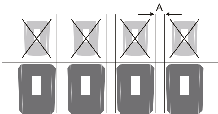
Bild 17: Väggmontering av flera växelriktare
