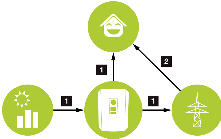
Bild 13: Styrning och fördelning av energiströmmarna
