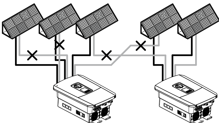
Bild 34: Felaktig koppling av solcellsgeneratorer
