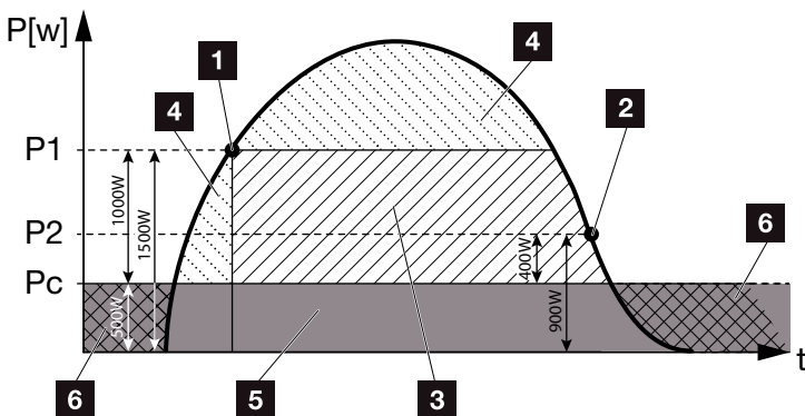
Bild 60: Kurva Dynamisk egenförbrukning (funktion 2)
