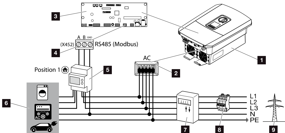
Bild 25: Anslutningsplan energimätare – husanslutning (position 1)
