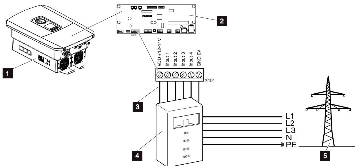
Bild 28: Rundstyrningsmottagare
