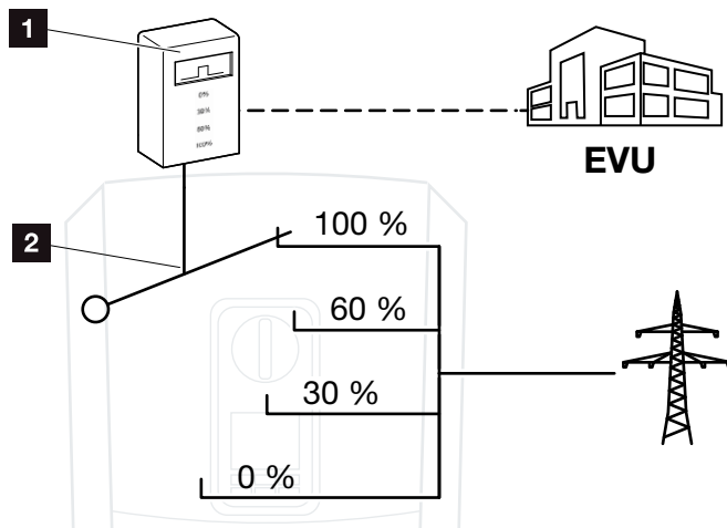
Bild 51: Aktiv effektstyrning med rundstyrningsmottagare
