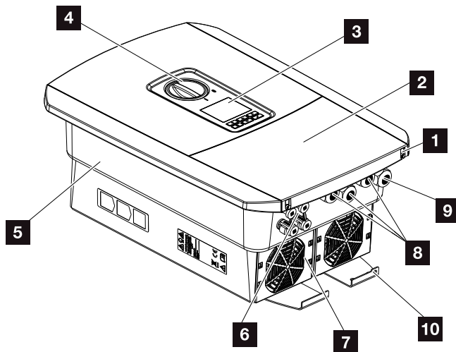
Bild 8: Växelriktare (utsida)
