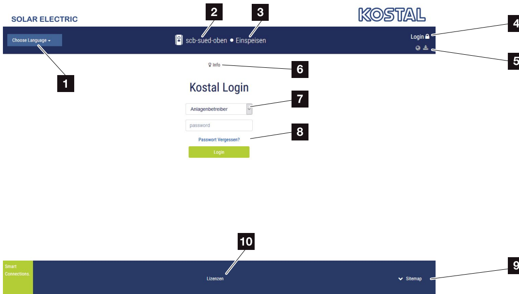
Bild 47: Webservern – startskärm
