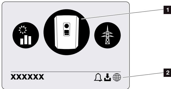
Bild 44: Huvudmenyns struktur
