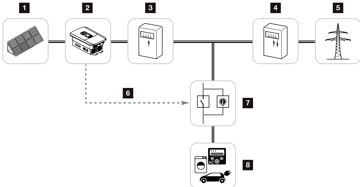
Bild 54: Konfiguration egenförbrukning
