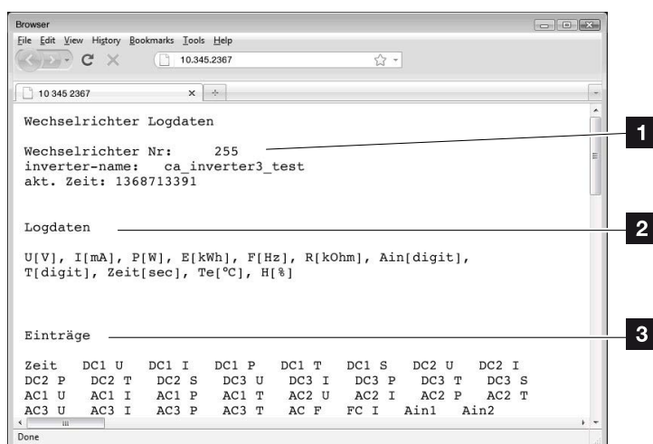
Fig. 48: Exemplo de ecrã "Ficheiro de registo"
