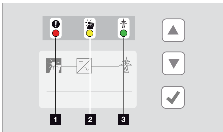
Fig. 41: LEDs no display do inversor
