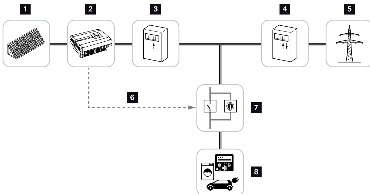
Fig. 53: Configuração do autoconsumo
