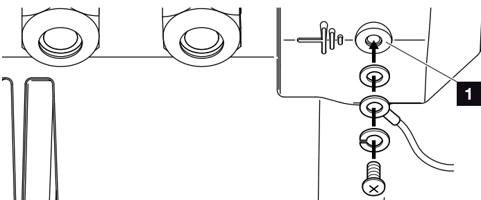
Fig. 24: Ligação PE específica do país
