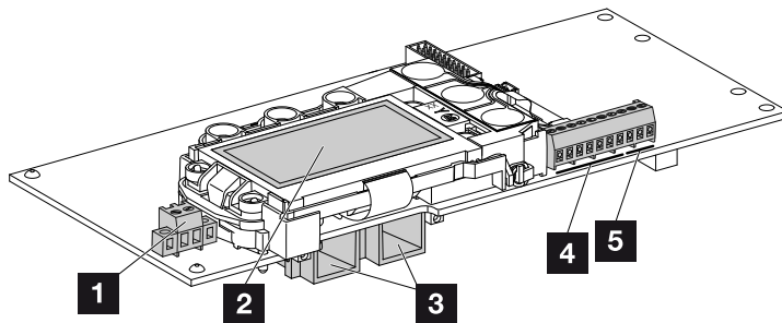
Fig. 14: Componentes da placa de comunicação
