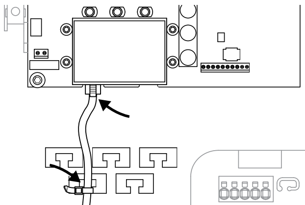
Fig. 35: Fixe o cabo no apoio do cabo
