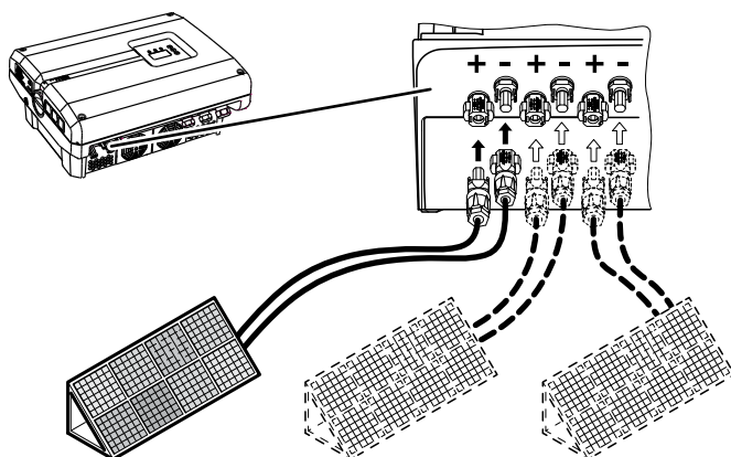
Fig. 30: Vista geral das ligações CC
