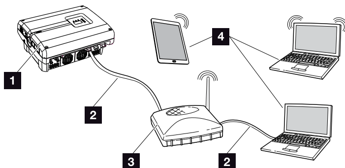
Fig. 47: Ligar o inversor ao computador através de um router
