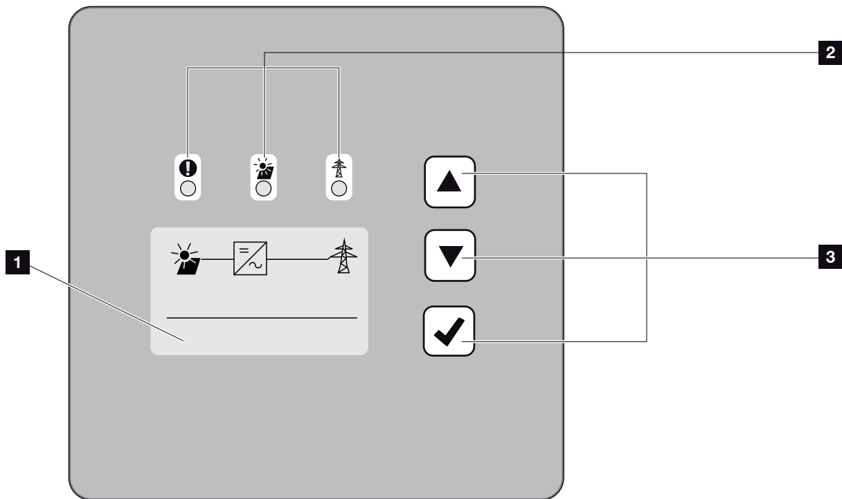
Fig. 15: Painel de controlo
