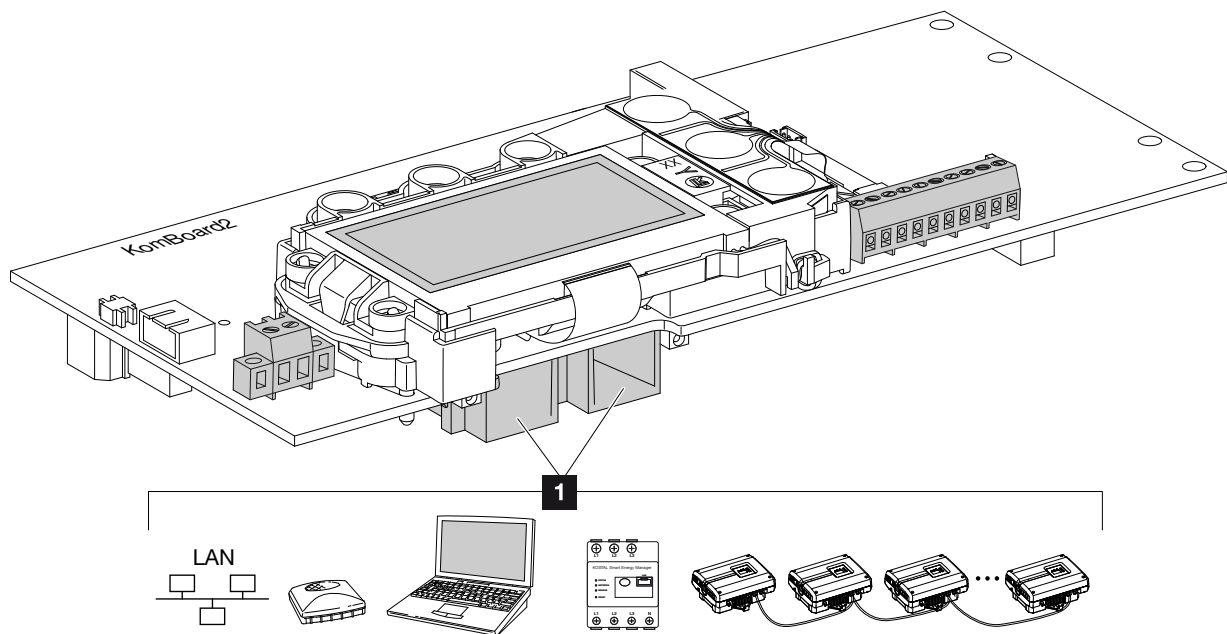
Fig. 34: Ocupação das tomadas de ligação
