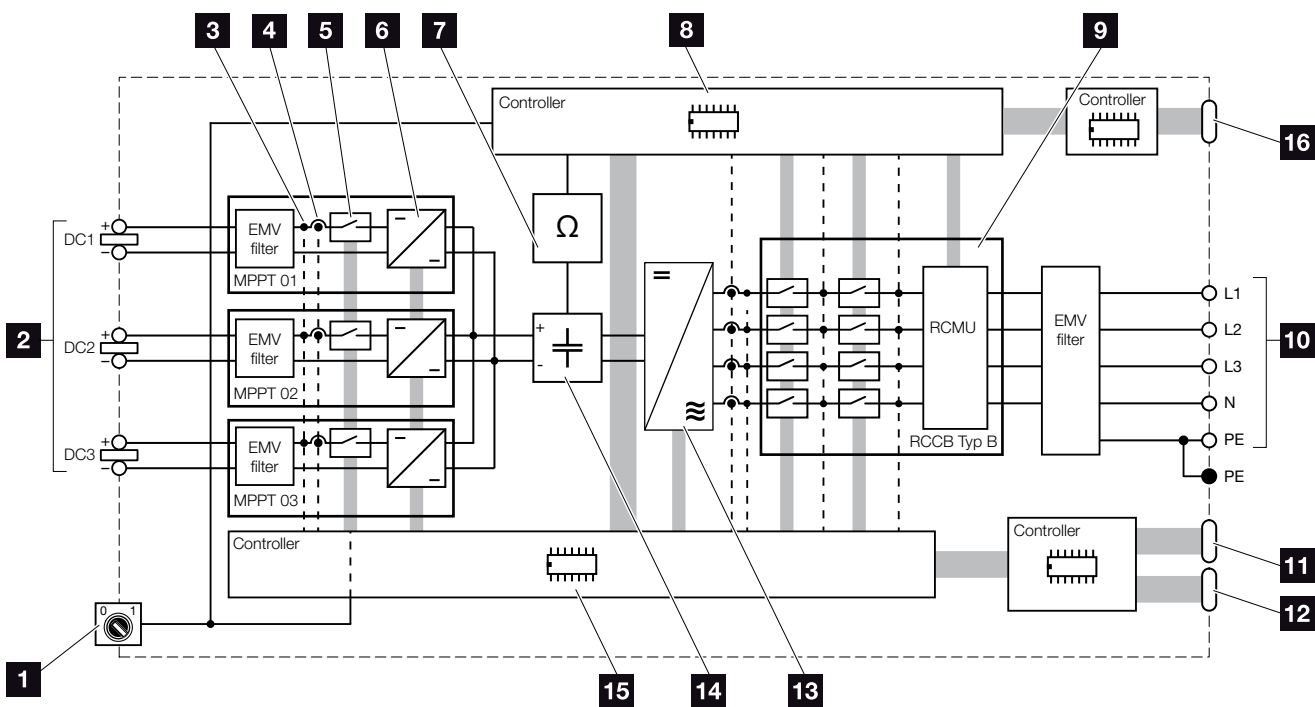
Fig. 65: Esquema de ligações
