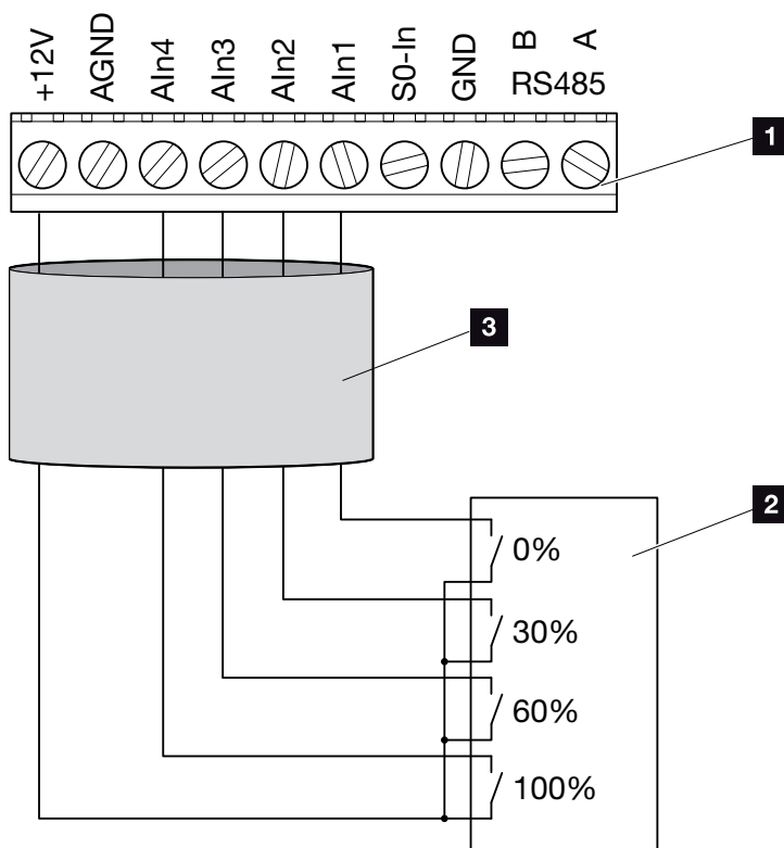
Fig. 52: Ligação do recetor de telecomando centralizado
