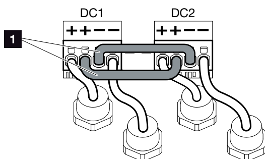
Fig. 28: Entradas 1 e 2 conectadas em paralelo
