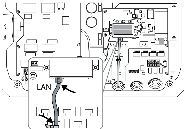
Fig. 67: Borne de ligação do contador de energia
