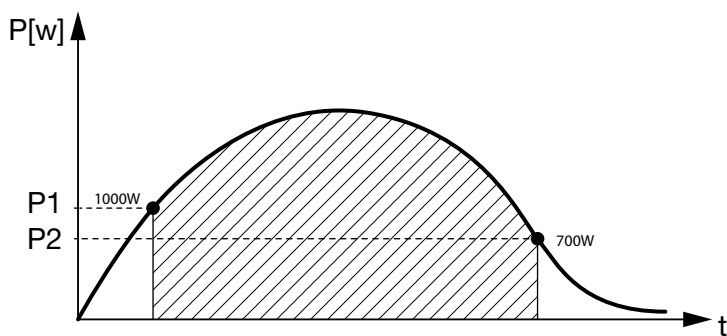
Fig. 57: Curva do autoconsumo (função 2) sem sensor
