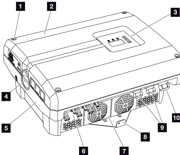
Fig. 9: Inversor PIKO
