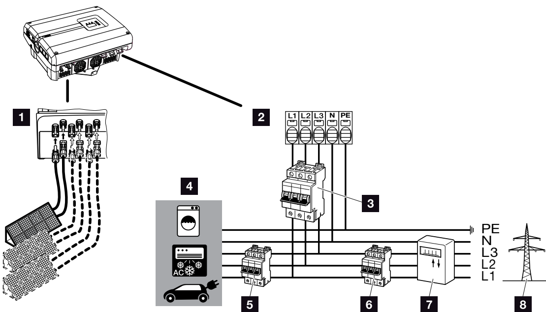
Fig. 21: Vista geral das ligações elétricas
