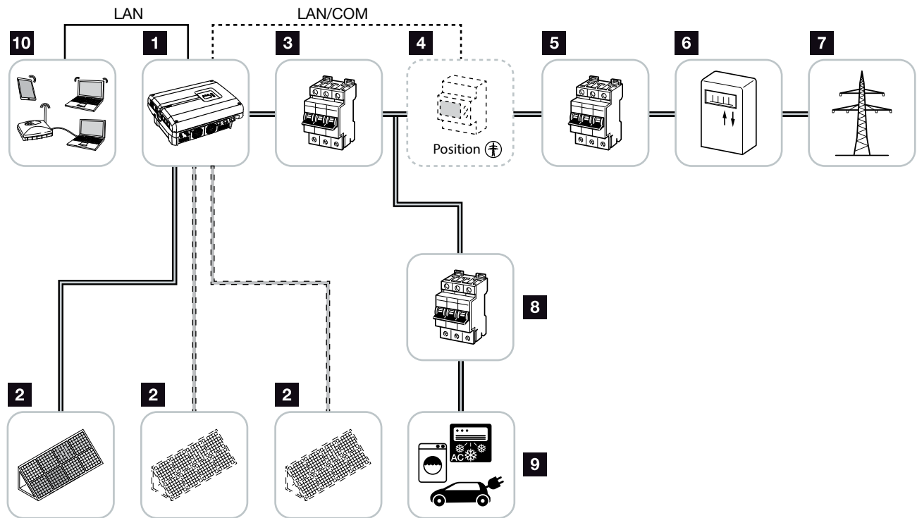
Fig. 8: Unidade fotovoltaica trifásica
