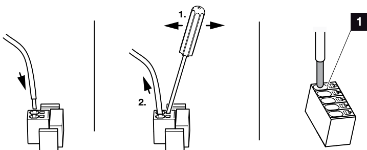
Fig. 23: Barra de bornes com mola de tração
