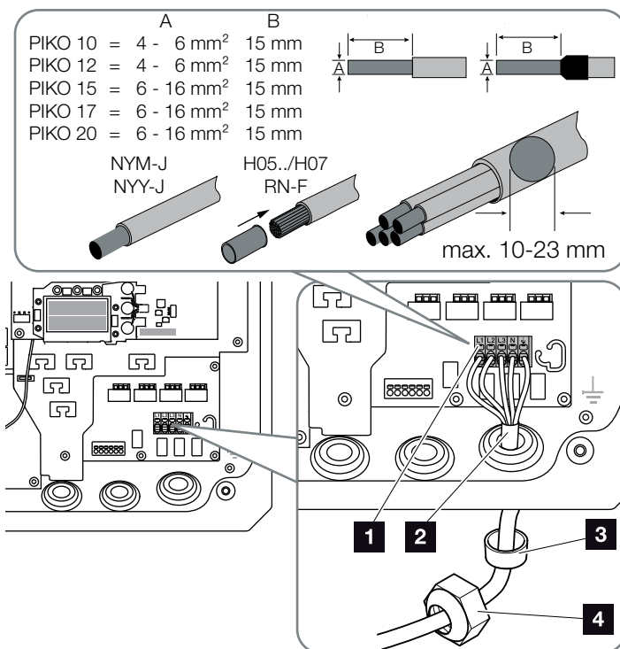
Fig. 22: Ligue o cabo de potência no inversor
