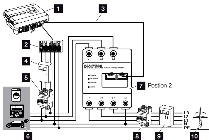
Fig. 66: Conexão do contador de energia
