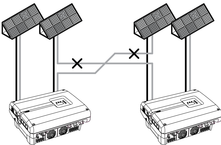
Fig. 29: Ligação incorreta dos geradores FV
