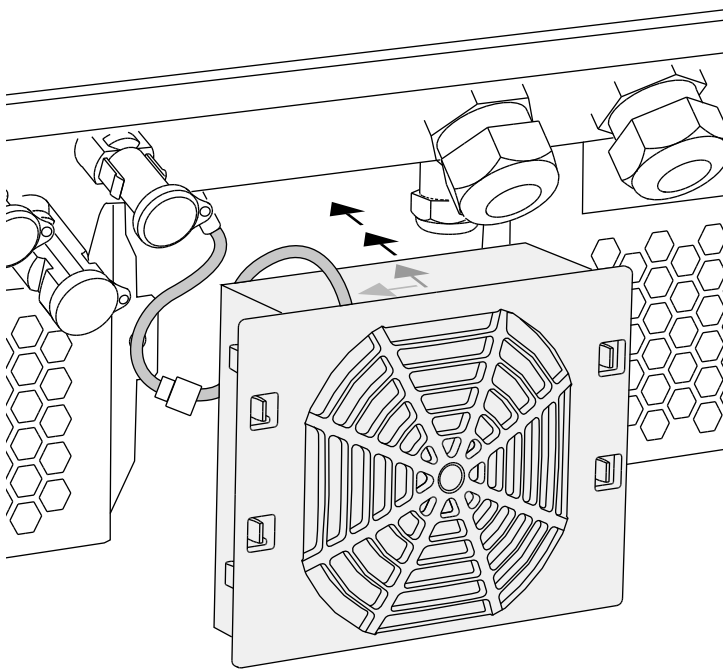
Fig. 64: Monte o ventilador
