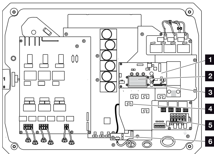
Fig. 13: Inversor PIKO 15-20 (vista interior)
