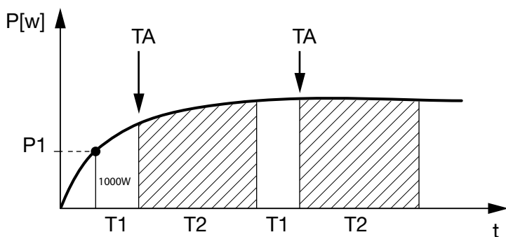
Fig. 56: Curva do autoconsumo (função 1) sem sensor de corrente
