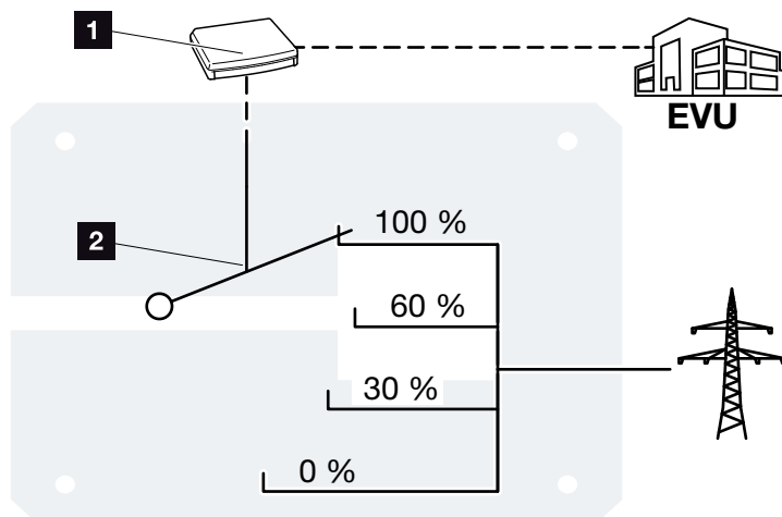
Fig. 50: Comando de potência ativa com um recetor de telecomando centralizado
