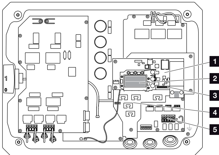
Fig. 12: Inversor PIKO 10-12 (vista interior)
