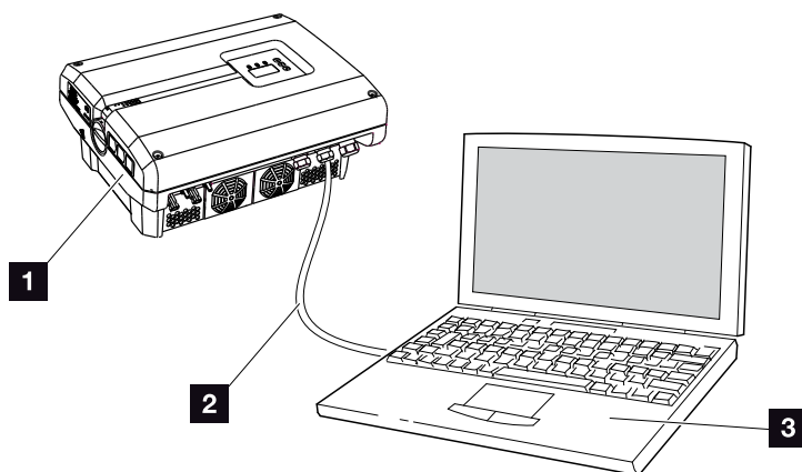
Fig. 46: Ligar o inversor diretamente ao computador
