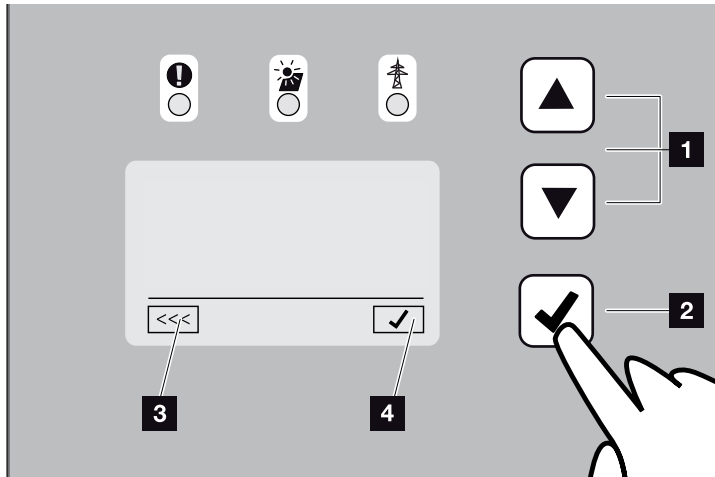
Fig. 39: Operação do display
