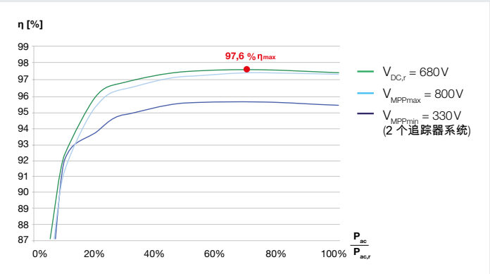
PIKO (比坤) 7.0 CN 的效率曲线
