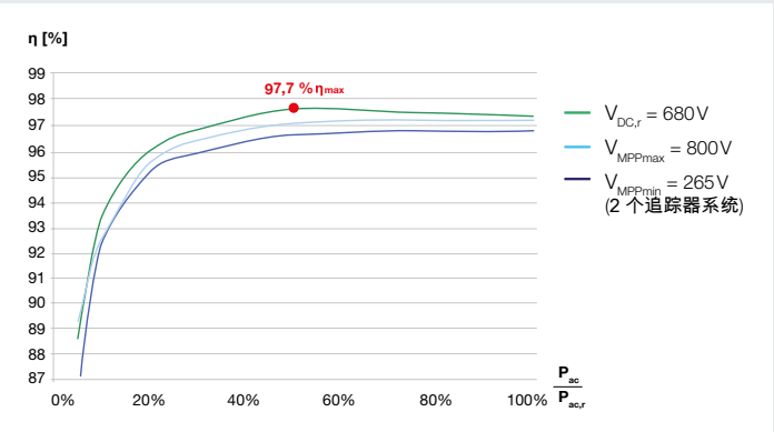
PIKO (比坤) 5.5 CN 的效率曲线
