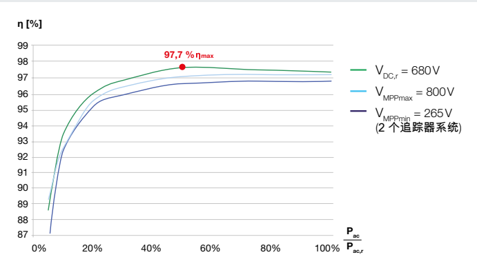
PIKO (比坤) 4.6 CN 的效率曲线
