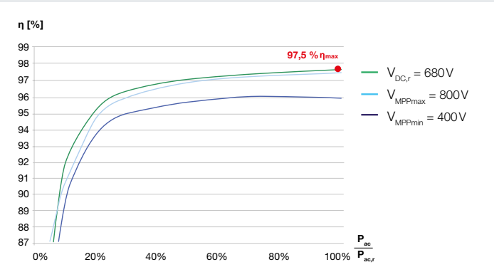
PIKO (比坤) 4.2 CN 的效率曲线
