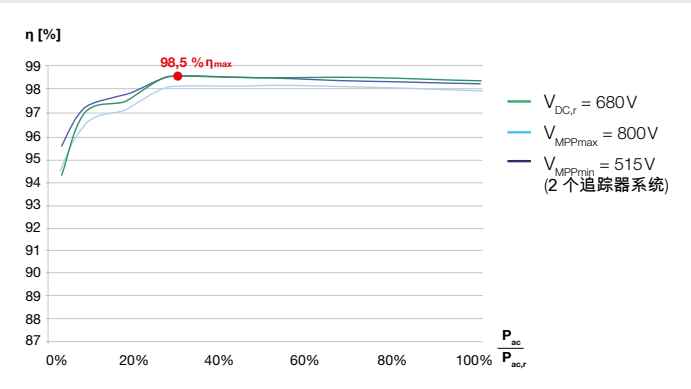
PIKO (比坤) 20 CN 的效率曲线
