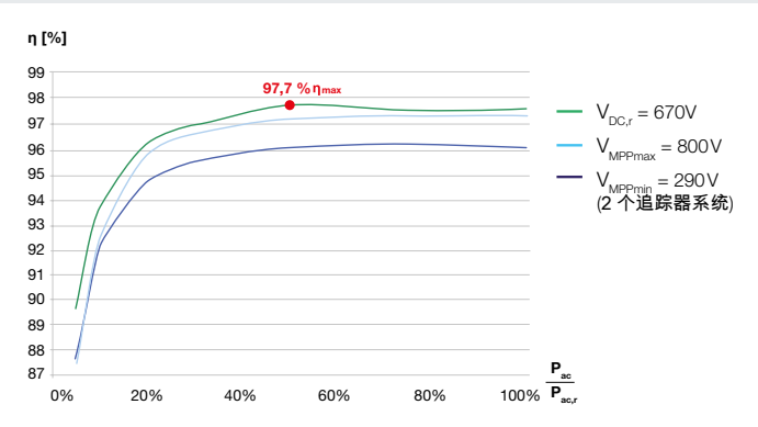
PIKO (比坤) 10 CN 的效率曲线
