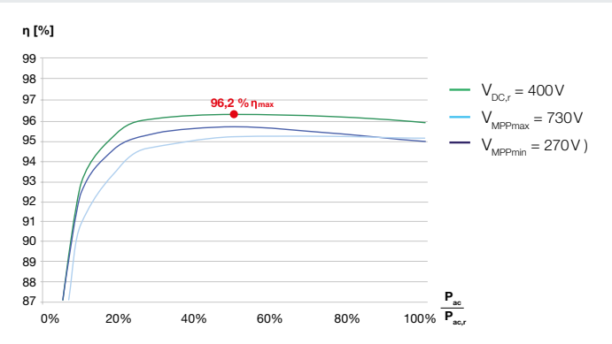
PIKO (比坤) 3.0 CN 的效率曲线
