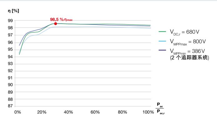
PIKO (比坤) 15 CN 的效率曲线
