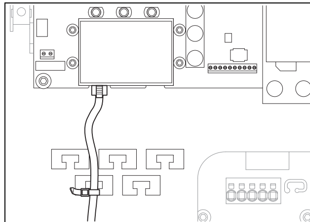
Abbildung 24: Kabel an Schutzblech befestigen
