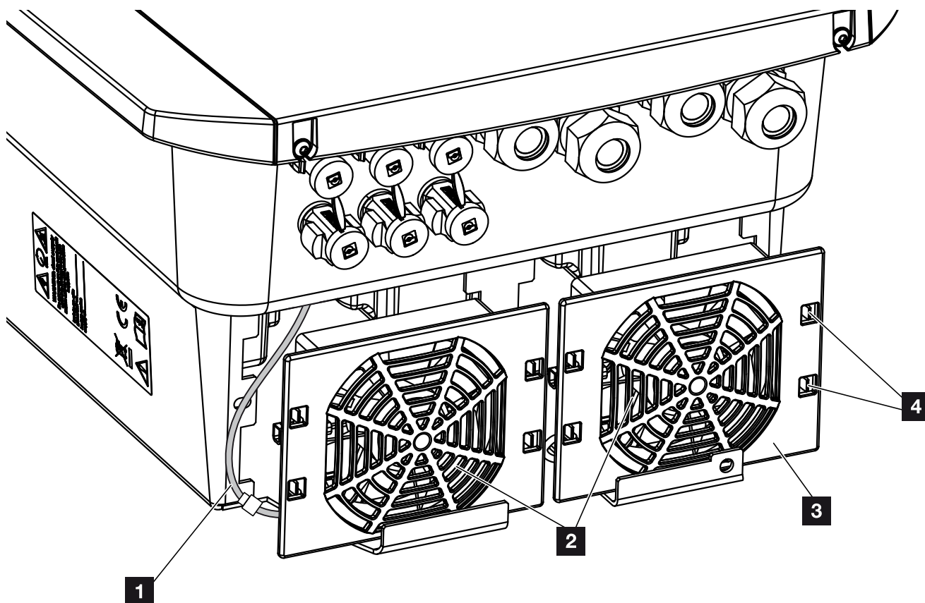
Afb. 72: Ventilator demontage overzicht
