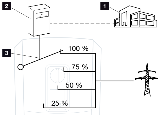
Afb. 60: Externe batterijregeling via digitale ingangen
