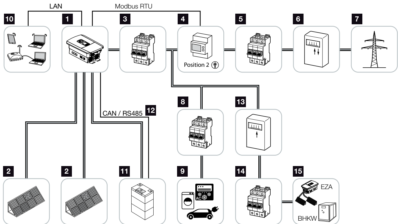
Afb. 9: Fotovoltaïsche installatie met AC-energieleverancier
