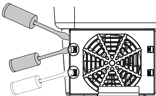
Afb. 74: Bevestigingslipjes losmaken
