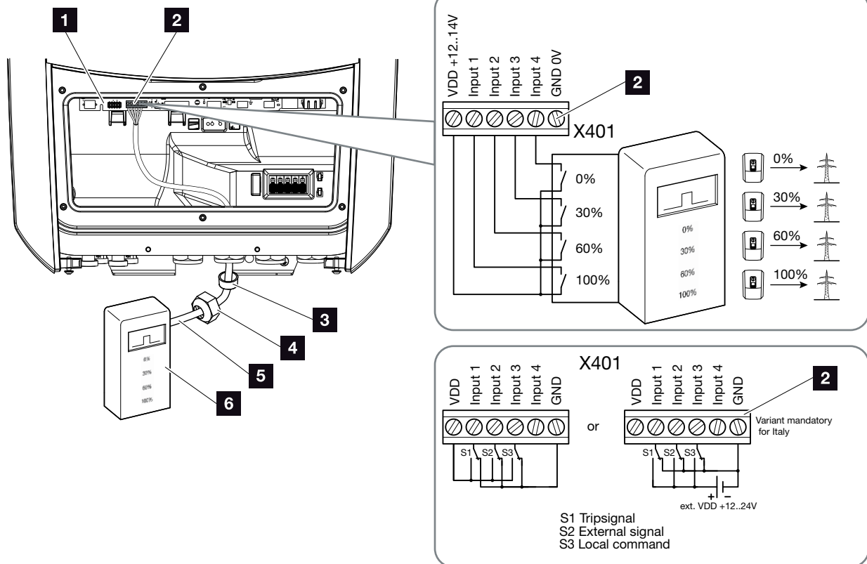
Afb. 31: Aansluiting rimpelspanningontvanger !
