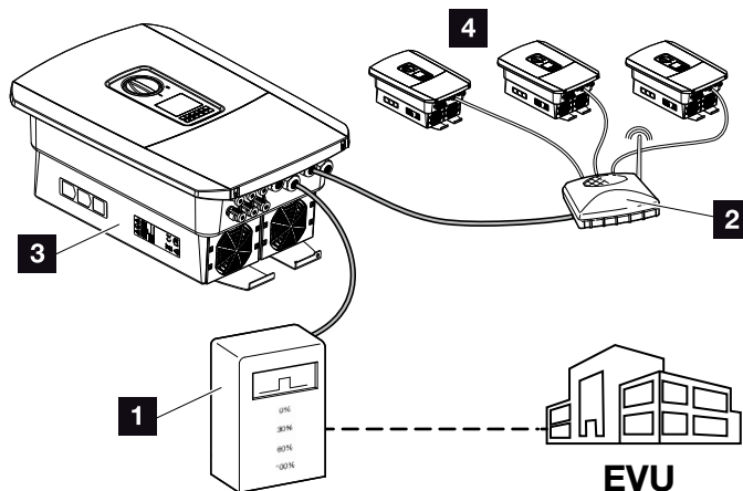
Afb. 62: Omvormer met rimpelspanningontvanger
