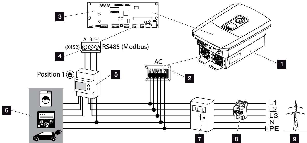
Afb. 27: Aansluitschema energieteller - huisaansluiting (positie 1)
