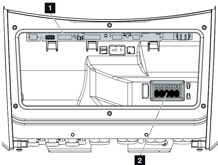
Afb. 13: Omvormer (binnenaanzicht)
