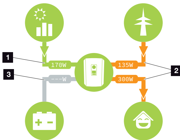
Afb. 54: Energie-stroomdiagram
