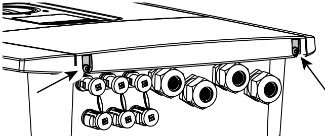
Afb. 21: Deksel wegnemen
