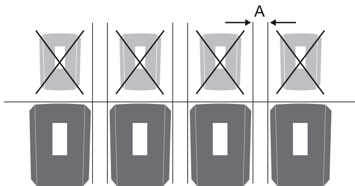
Afb. 19: Wandmontage van meerdere omvormers
