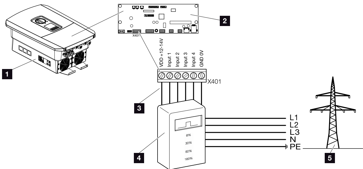
Afb. 30: Rimpelspanningontvanger
