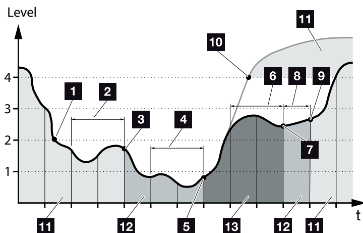
Afb. 55: Automatische modus
