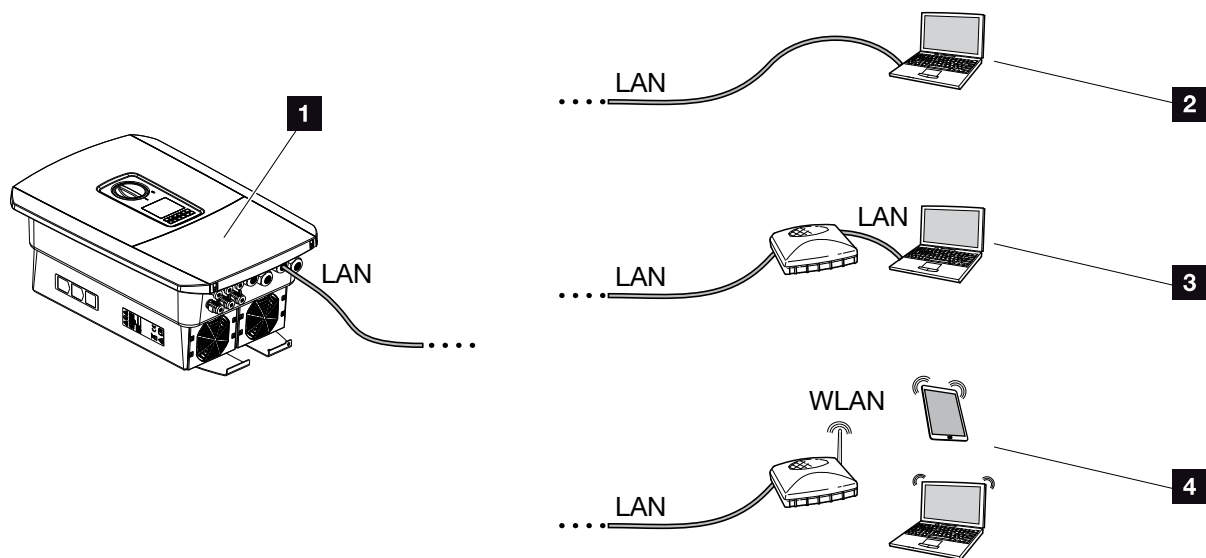
Afb. 50: Verbinding van computer met de omvormer
