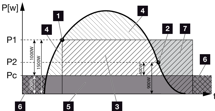
Afb. 70: Curve dynamisch eigenverbruik (functie 2)
