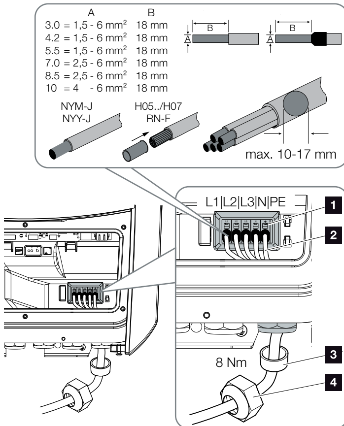
Afb. 23: Voedingsleiding op de omvormer aansluiten
