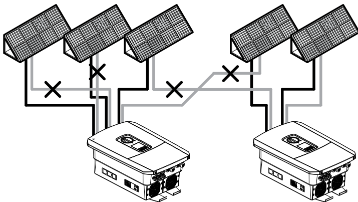
Afb. 39: Foutieve bedrading fotonvoltaïsche generatoren
