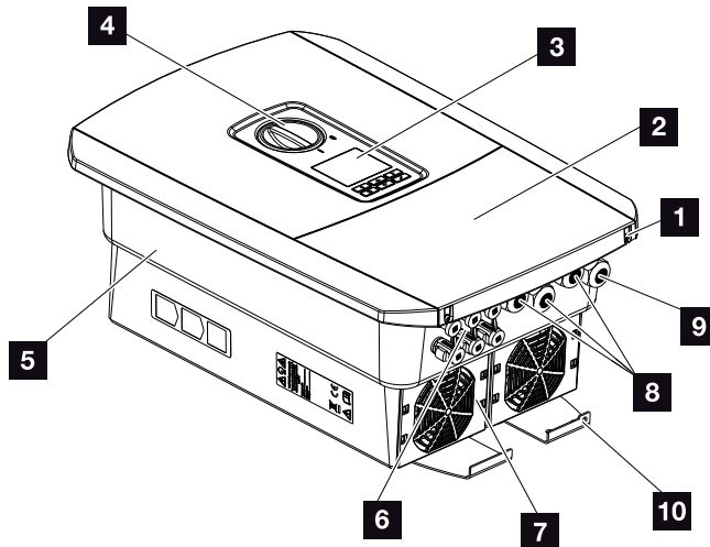
Afb. 10: Omvormer (buitenaanzicht)
