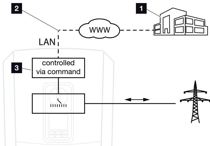
Afb. 59: Externe batterijregeling via Modbus (TCP)
