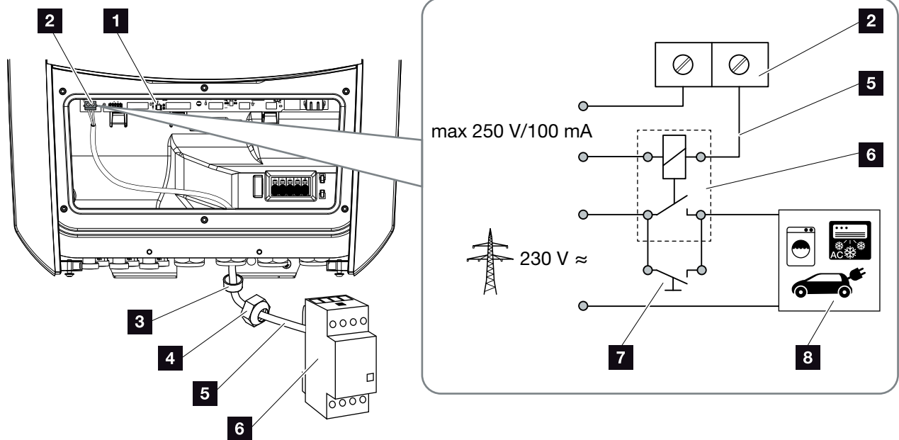
Afb. 65: Elektrische aansluiting eigenverbruiksregeling
