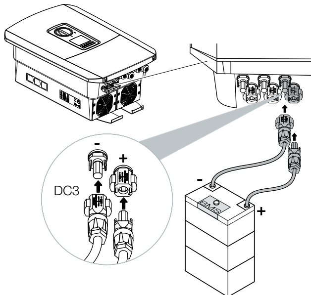
Afb. 38: Overzicht DC-aansluiting batterij
