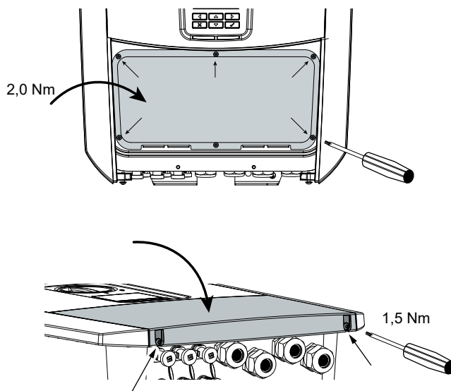
Afb. 37: Omvormer sluiten
