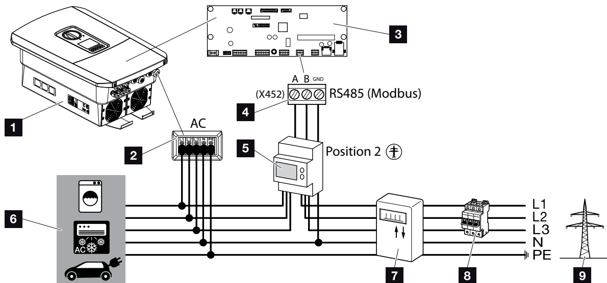
Afb. 28: Aansluitschema energiemeter - netaansluiting (positie 2)
