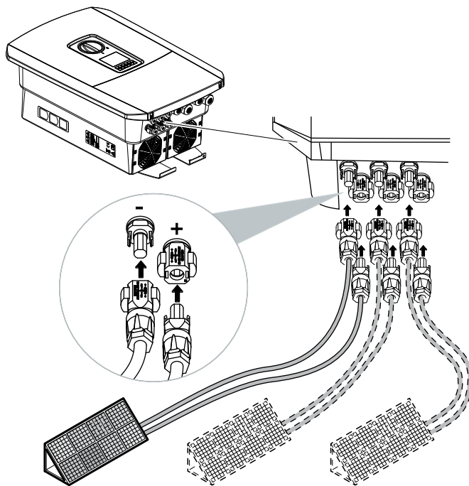
Afb. 40: Overzicht DC-aansluitingen
