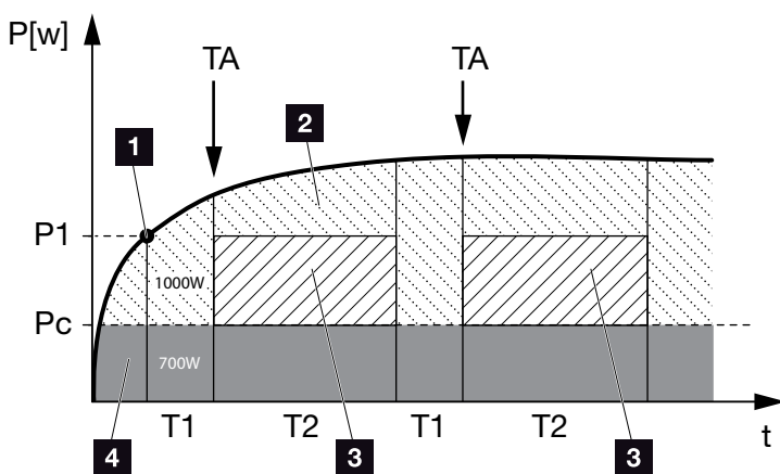
Afb. 68: Curve dynamisch eigenverbruik (functie 1)
