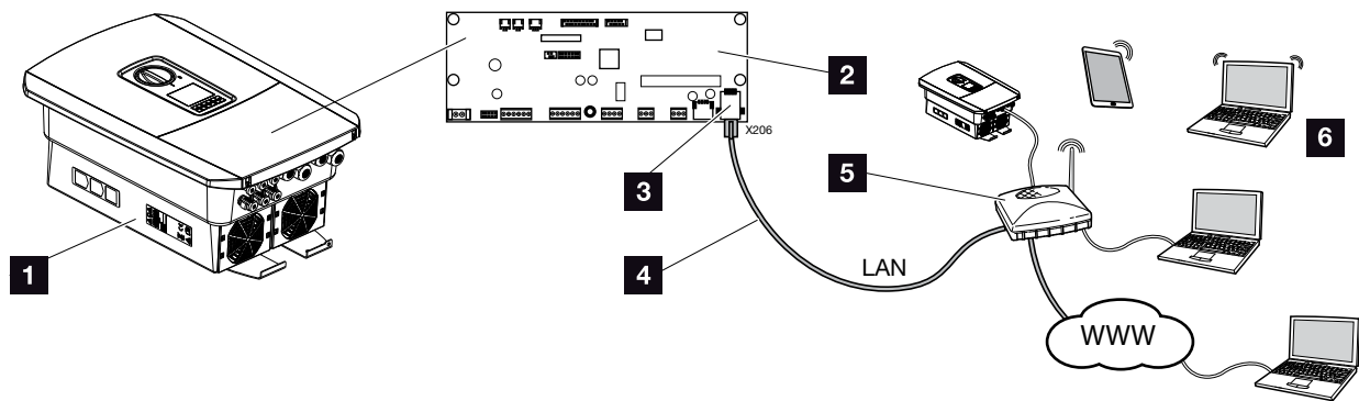
Afb. 33: Aansluiting communicatie
