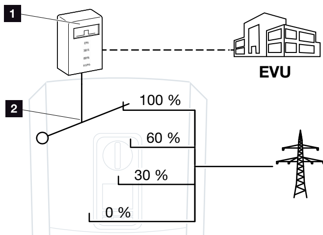
Afb. 61: Vermogensbesturing met rimpelspanningontvanger
