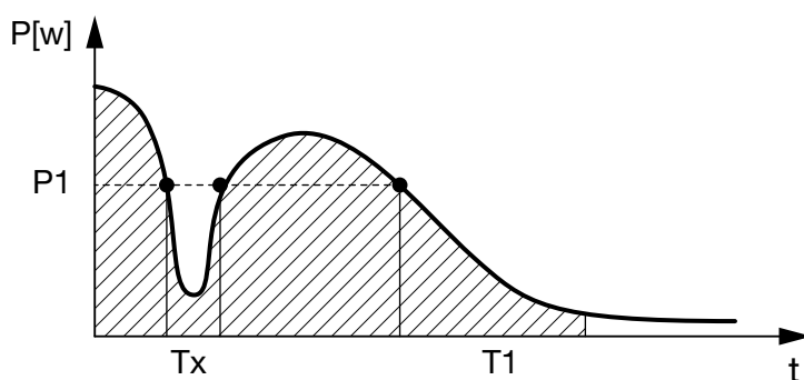
Afb. 71: Curve vertraging bij vermogensverlies/storing
