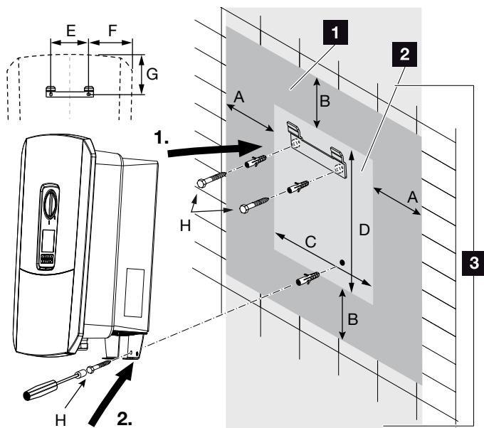
Afb. 18: Wandmontage m.b.v. wandhouder
