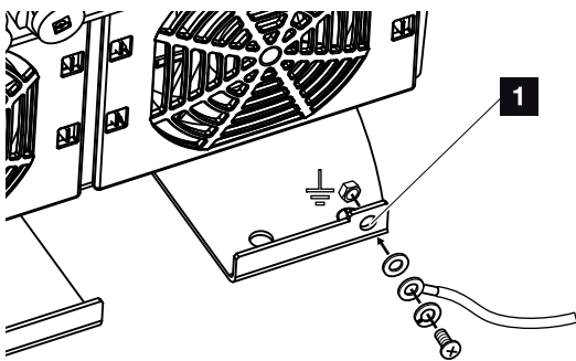
Afb. 25: Landspecifieke PE-aansluiting buiten
