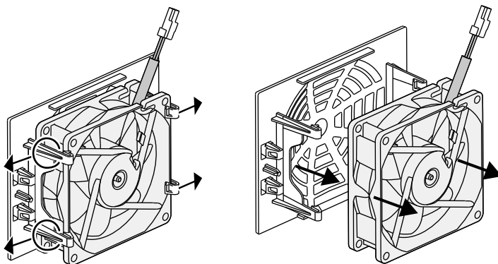
Afb. 76: Demontage ventilatorrooster
