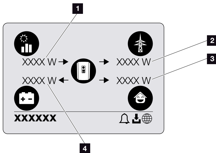
Afb. 48: Vermogensstroomdiagram
