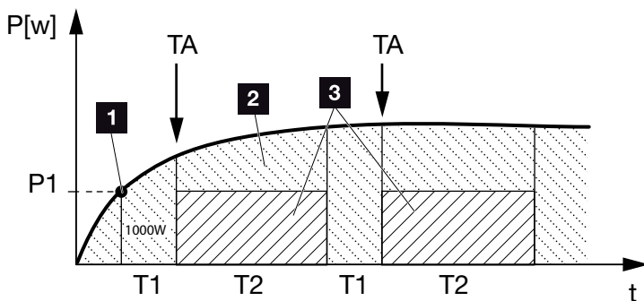
Afb. 67: Curve eigenverbruik (functie 1)
