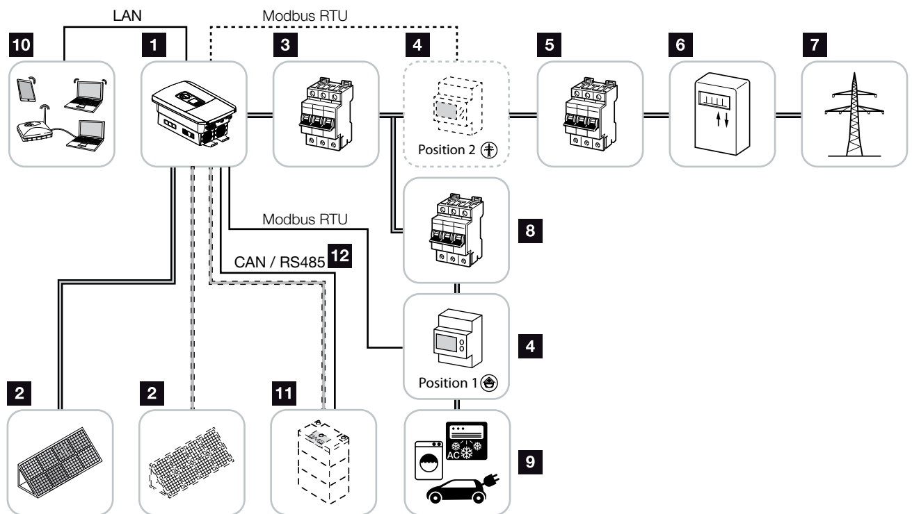
Afb. 8: Fotovoltaïsche installatie met PV en batterijaansluiting
