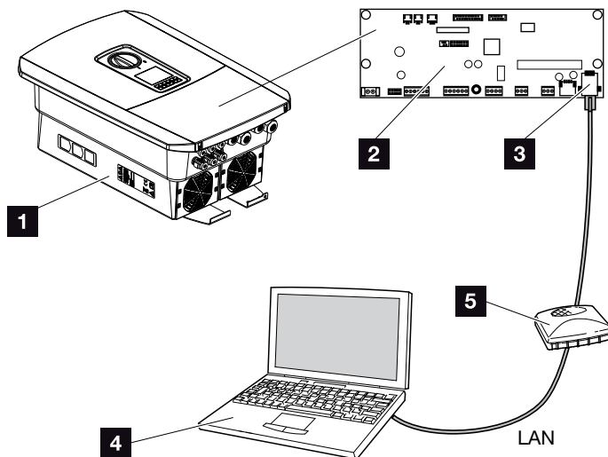
Afb. 51: Omvormer en computer met ethernetkabel verbinden
