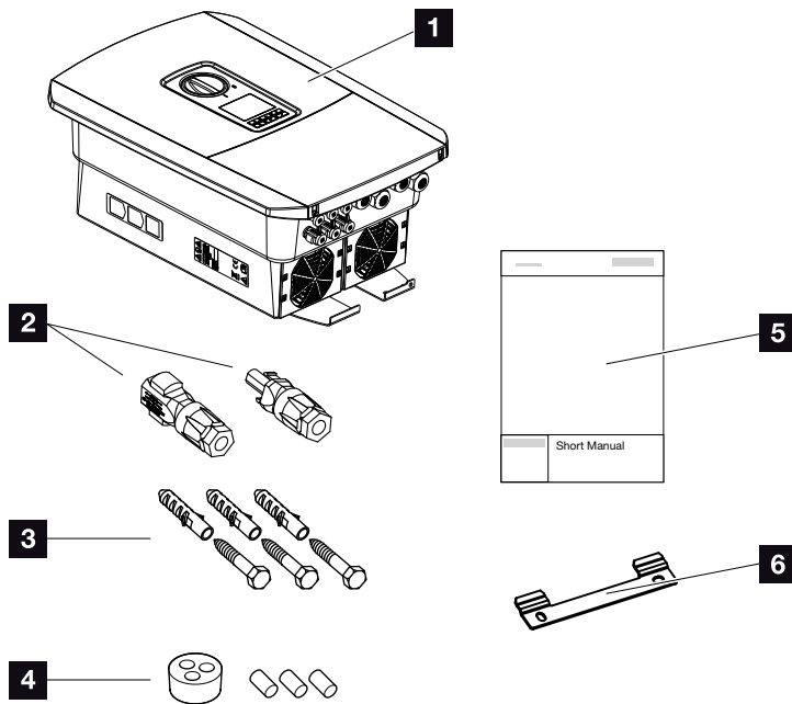
Afb. 17: Leveringsomvang
