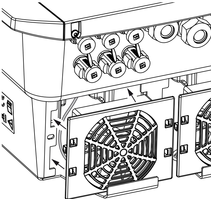
Afb. 77: Ventilatormontage
