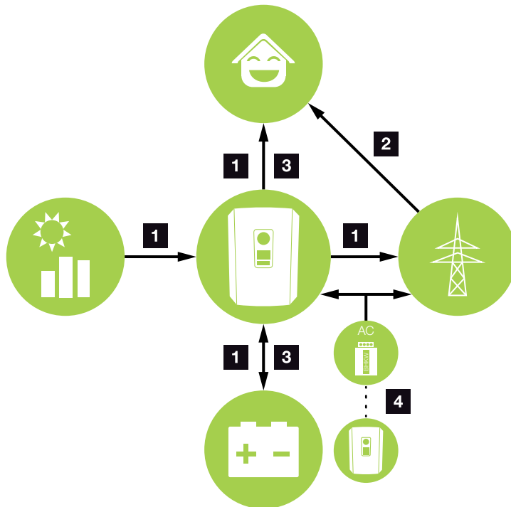
Afb. 15: Regeling en verdeling van de energiestromen
