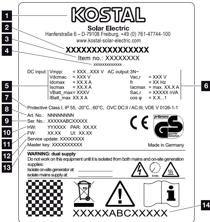
Afb. 79: Typeplaatje
