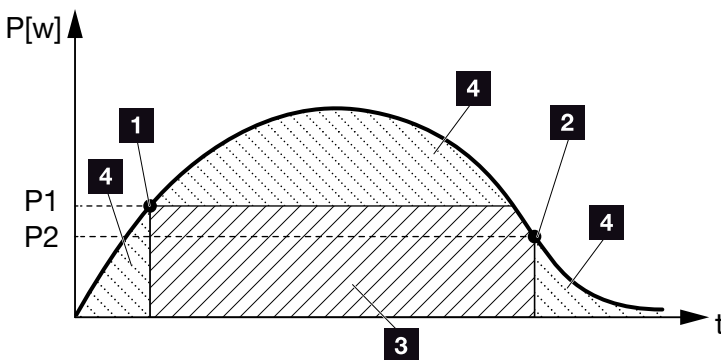
Afb. 69: Curve eigenverbruik (functie 2)
