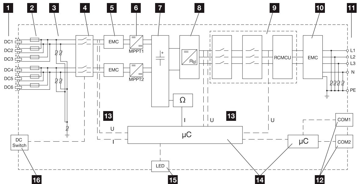
Blokové schéma 30
