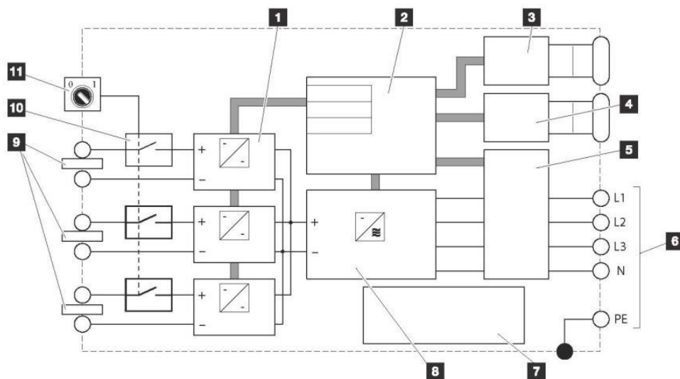
Abb. 68: Blockschaltbild
