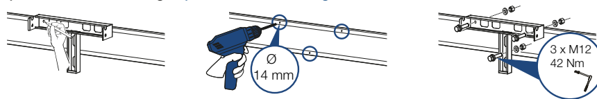
Optional - Frame mounting / Optional - Gestellmontage
